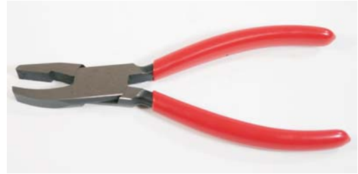
32 120 00 KNIPEX Brech- und Kröselzange, 160 mm Länge, 10 mm Backenbreite ölgehärtete Backen, ummantelter Griff Breaking and grozing pliers, 160 mm l., 10 mm jaw width, oil tempered jaw, coated grip
